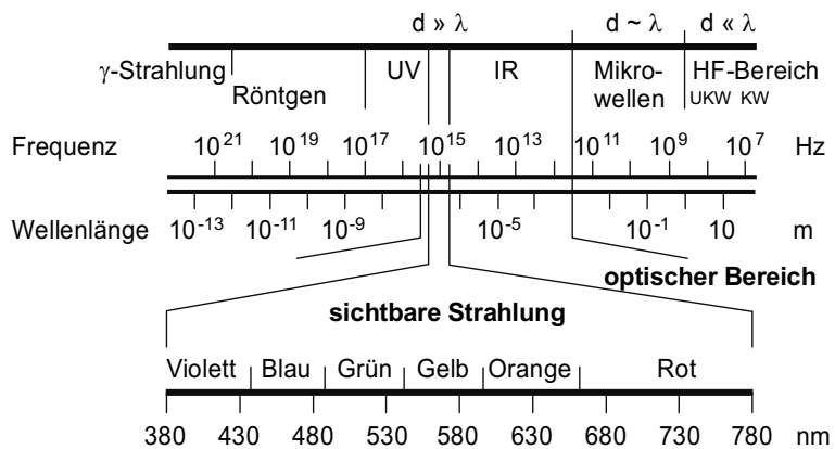
Bild 1.1 Frequenz- und Wellenlängenbereiche der elektromagnetischen Strahlung
