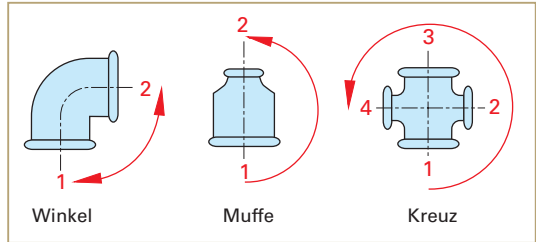
Bild 1: Reihenfolge der Abgangsbezeichnungen bei Fittings
