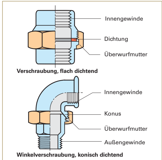
Bild 2: Verschraubungen
