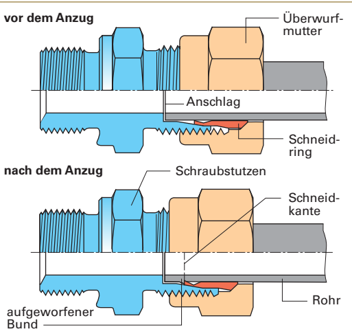
Bild 1: Schneidringverschraubung
