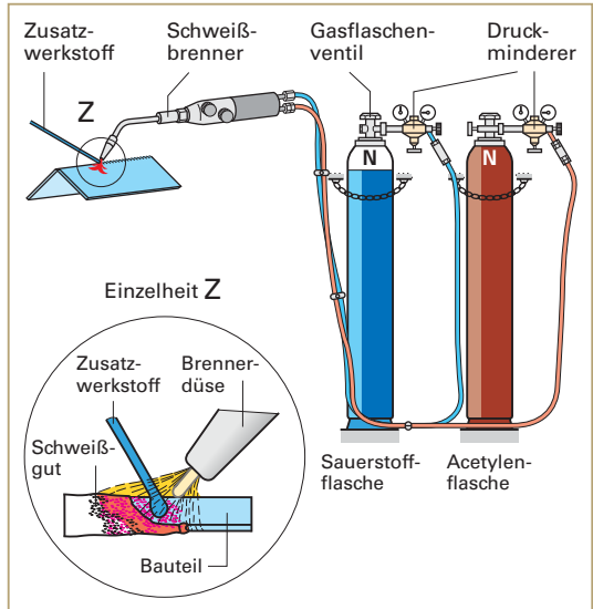
Bild 1: Gasschmelzschweißen
