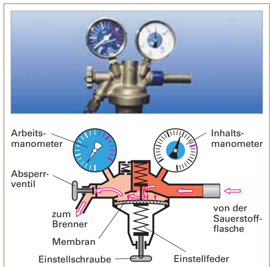
Bild 2: Druckminderer
