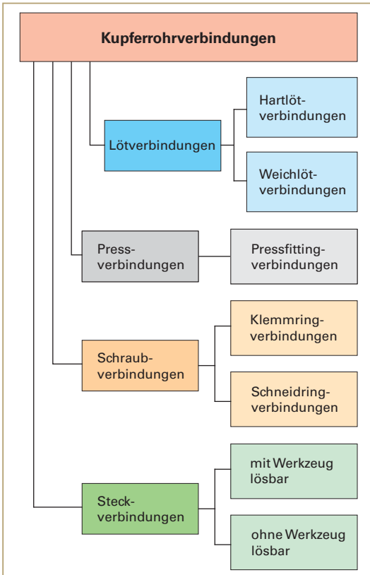
Bild 2: Kupferrohrverbindungen (Übersicht)
