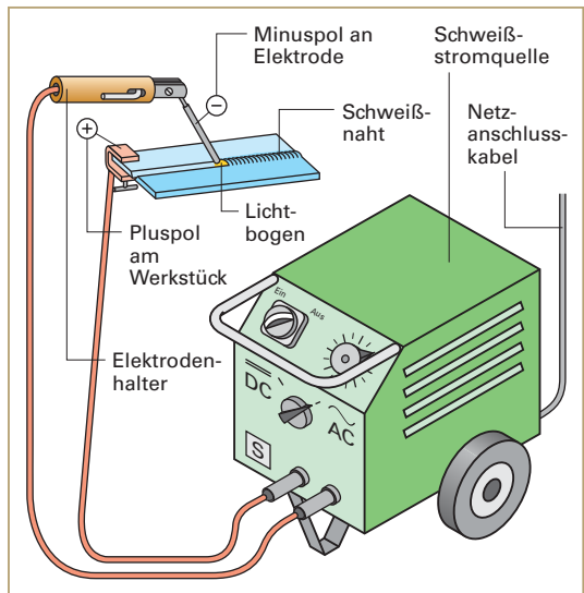
Bild 3: Lichtbogenhandschweißen
