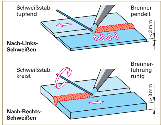
Bild 1: Schweißmethoden
