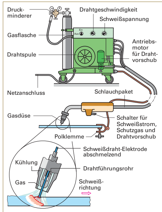
Bild 1: MAG-Schweißanlage
