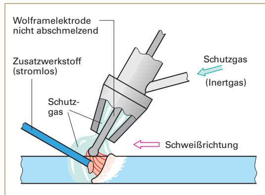
Bild 2: WIG-Schweißen
