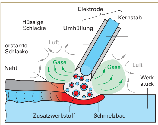
Bild 2: Abbrenverhalten der Elektrode beim Lichtbogenhandschweißen
