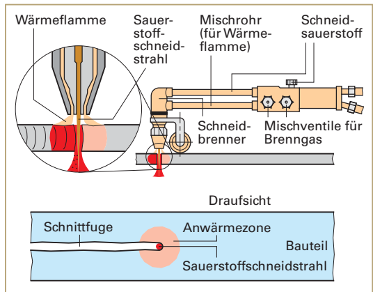
Bild 2: Brennschneiden
