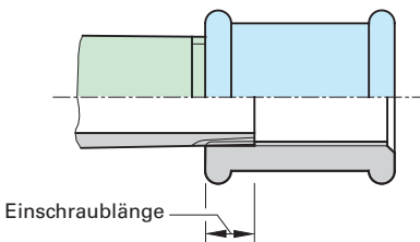
Bild 1: Gewindeverbindung
