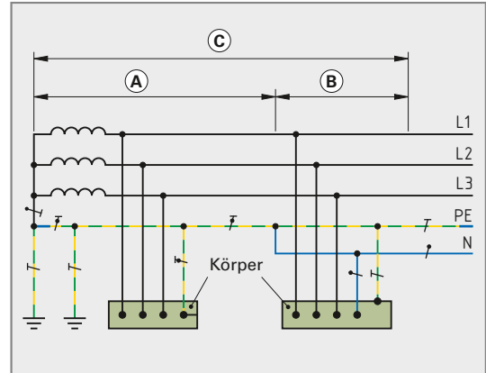
Bild 1: Verteilungssystem zu Frage 2
