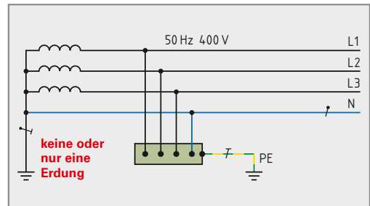
Bild 2: Verteilungssystem zu Frage 3
