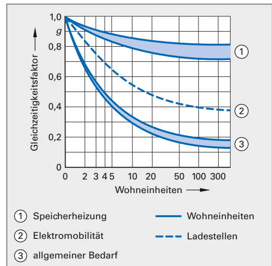
Bild 2: Gleichzeitigkeitsfaktoren bei Wohnanlagen
