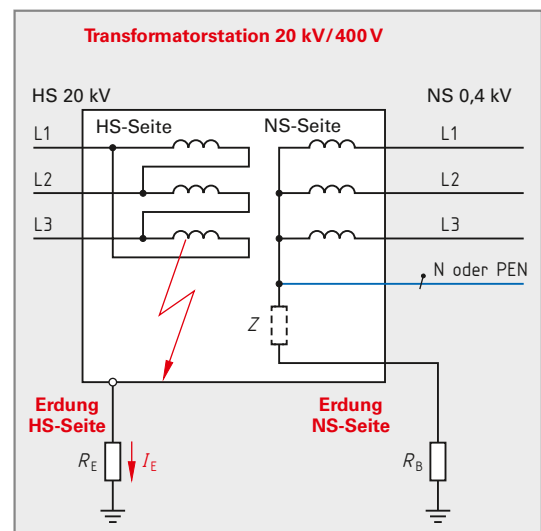
Bild 2: Transformatorstation für Übergang Hochspannungsnetz zu Niederspannungsnetz
