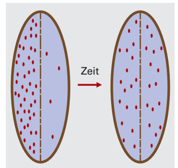
3 Diffusion durch eine semipermeablen Membran
